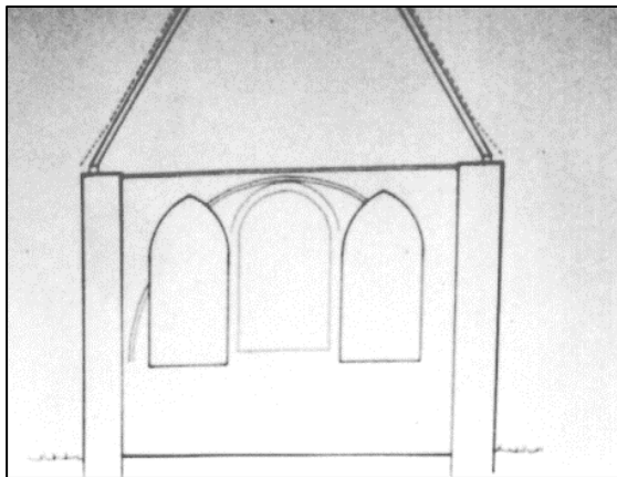
15.4 De Westmuur Historische bouwsporen
